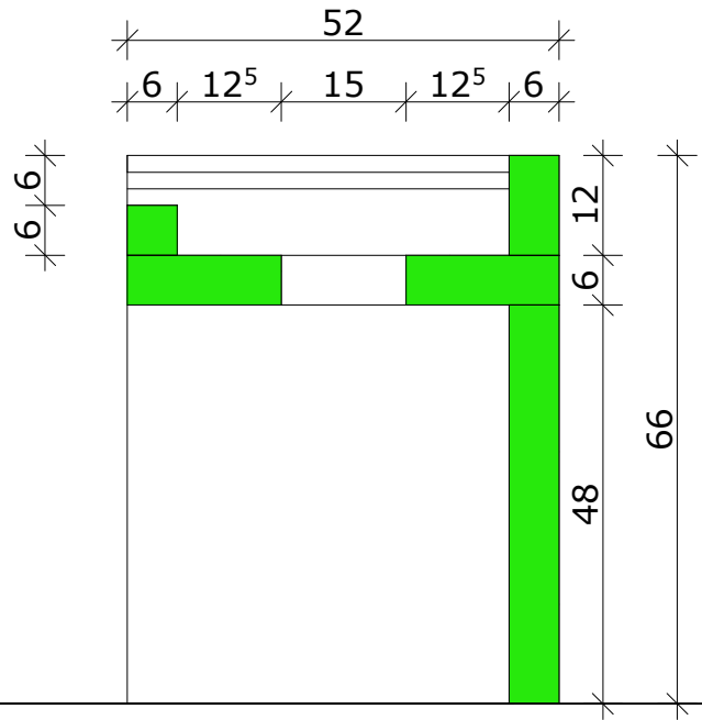
SCHNITT F-F
