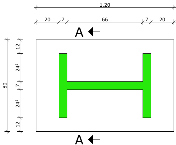
GRUNDRISS
